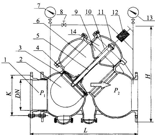
图 A. 0. 2-10 先导式稳压减压阀(Y形,带有过滤网和伸缩法兰)
