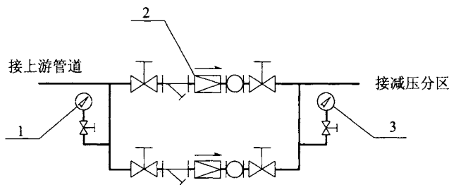
图 3.2.18-1 减压阀并联阀组水平布置示意图
