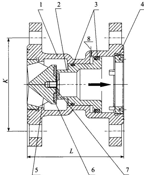
图 A. 0. 1-2 法兰连接比例式减压阀结构示意图
