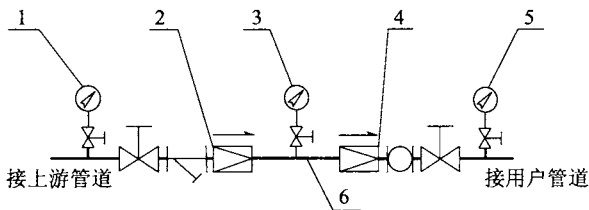
图 3.2.19-1 单阀组串联减压布置示意图
