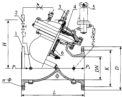
图 A.0.2-9 先导式稳压减压阀(Y形)
