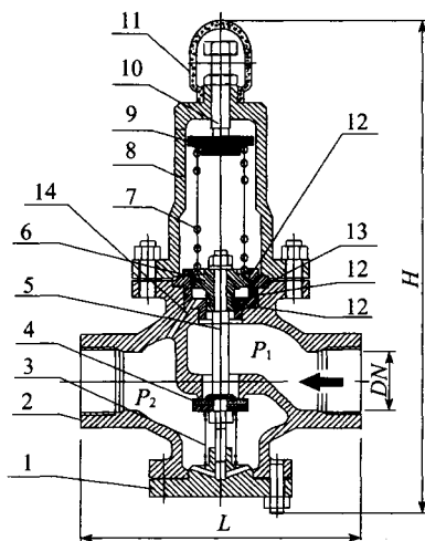
图 A. 0. 2-1 直接作用式稳压减压阀结构 I 型
