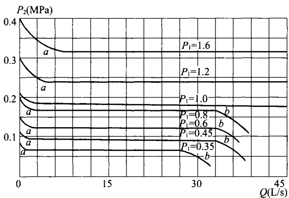
图 10 DN65(4 : 1)比例式减压阀流量-压力特性曲线
