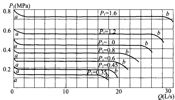
图 8 DN65(2 : 1)比例式减压阀流量-压力特性曲线
