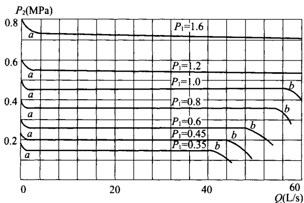
图 13 DN150(2 : 1)比例式减压阀流量-压力特性曲线
