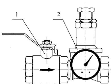
图 15 差压式可调减压阀组合装置示意
