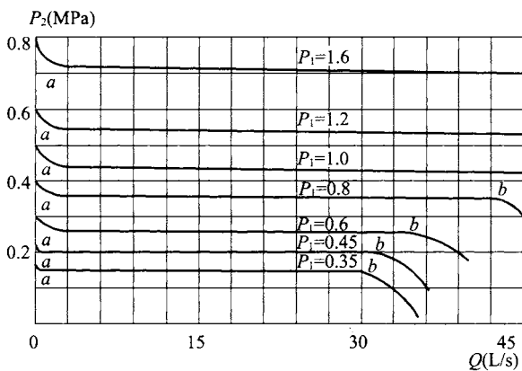
图 12 DN100(2:1)比例式减压阀流量-压力特性曲线
