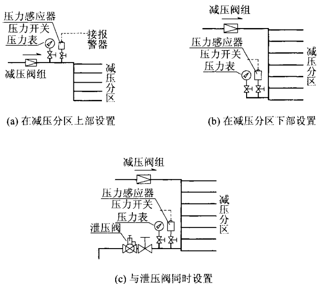
图 5 超压报警装置的压力感应器设置示意
