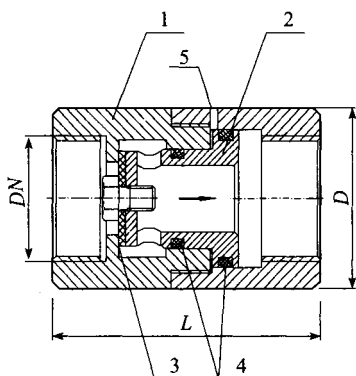
图 A.0.1-1 螺纹连接比例式减压阀结构示意图
