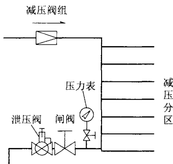
图 4 自动泄压阀设置示意
