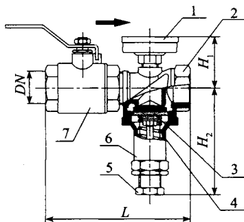
图 A.0.3 自动泄压阀组合装置结构示意图
