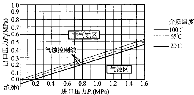
图 3.3.3 单级减压阀气蚀控制图
