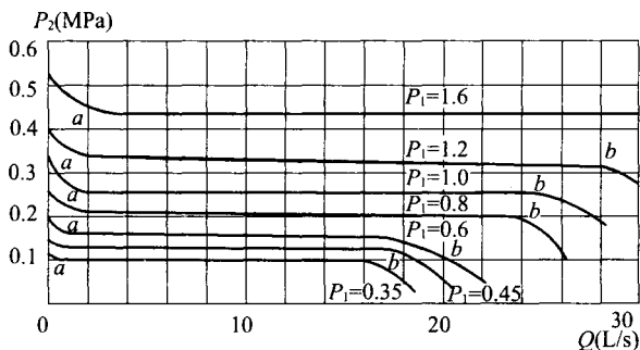
图 9 DN65(3 : 1)比例式减压阀流量-压力特性曲线
