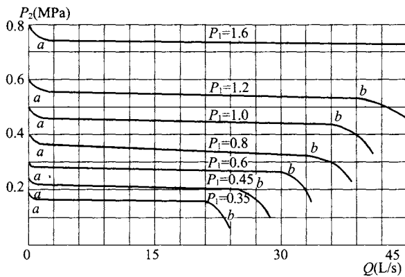
图 11 DN80(2:1)比例式减压阀流量-压力特性曲线
