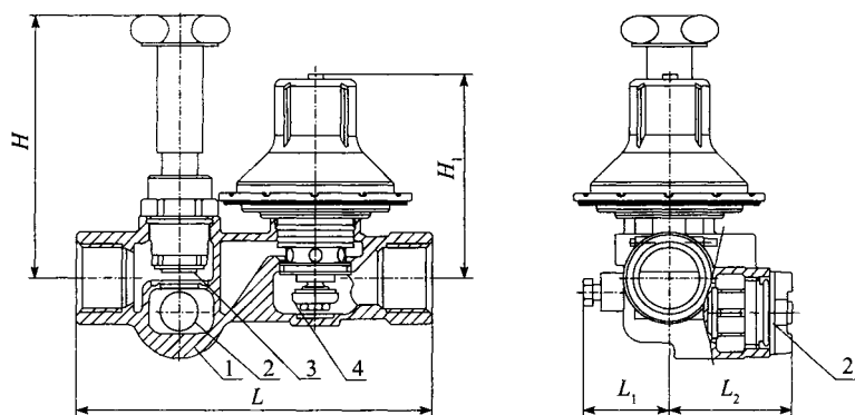
图 A.0.2-3 直接作用式稳压减压阀结构Ⅲ型(分户减压阀)
