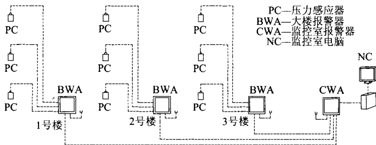
图 6 超压报警装置布置示意
