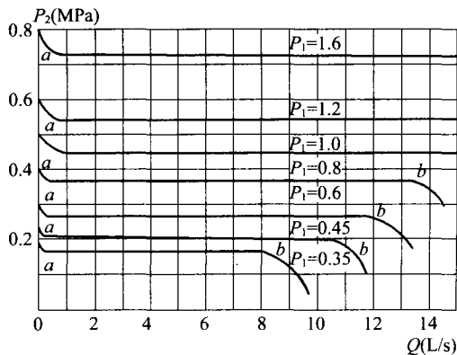
图 7 DN50(2:1)比例式减压阀流量-压力特性曲线
