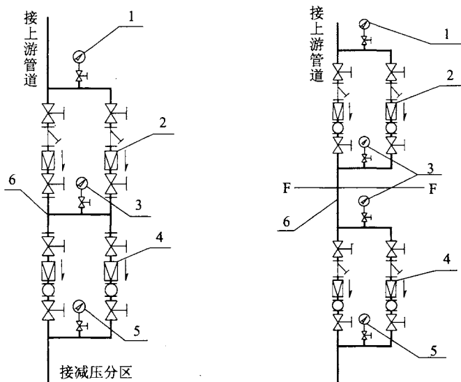
(a) 减压阀串联阀组（同层布置）
