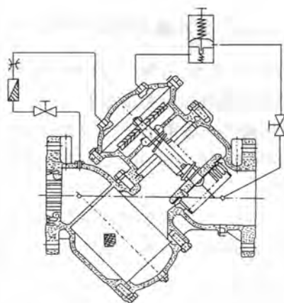
图 2 防气蚀大压差减压阀结构图
