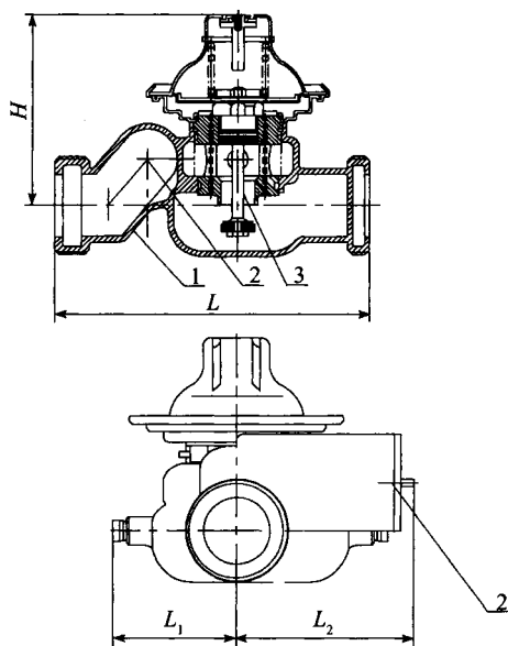
图 A. 0. 2-5 直接作用式稳压减压阀结构 V 型(分户减压阀)
