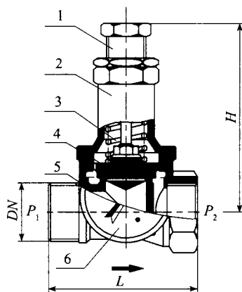
图 A. 0. 2-11 直接作用式差压减压阀结构尺寸
