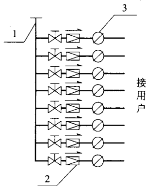
图 3.2.1-2 直接作用式稳压减压阀设置示意图
