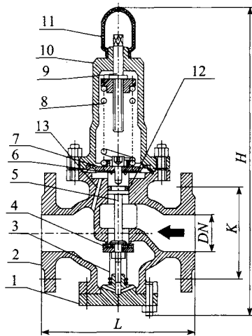
图 A. 0. 2-6 直接作用式稳压减压阀(法兰连接)结构图
