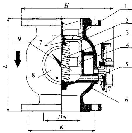
图 A.0.2-8 先导式稳压减压阀(立式)
