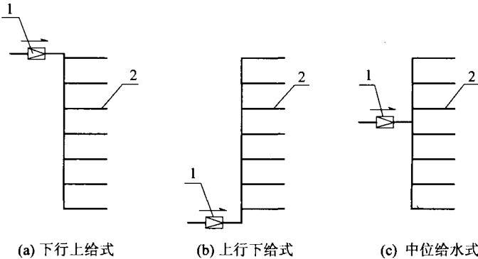
图1 减压分区进水方式示意图
