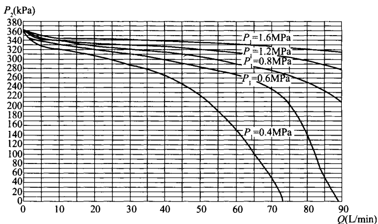
图 14 直接作用式稳压减压阀(MS、MW-20A 型)流量-压力特性曲线
