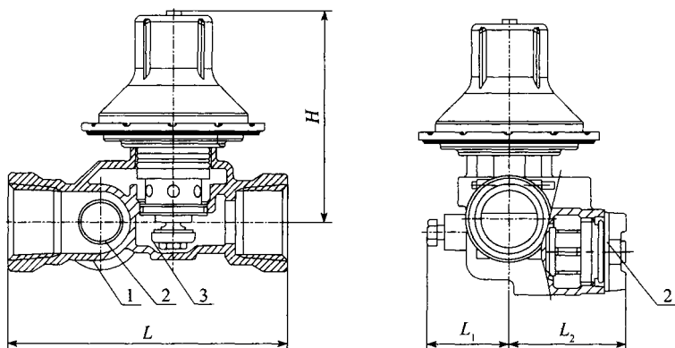
图 A.0.2-4 直接作用式稳压减压阀结构Ⅳ型(分户减压阀)
