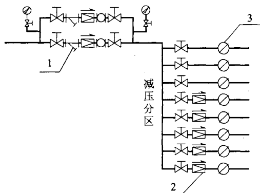
图 3.2.1-1 直接作用式差压减压阀设置示意图
