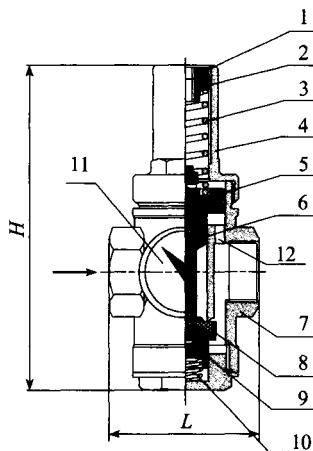
图 A. 0. 2-2 直接作用式稳压减压阀结构 II 型
