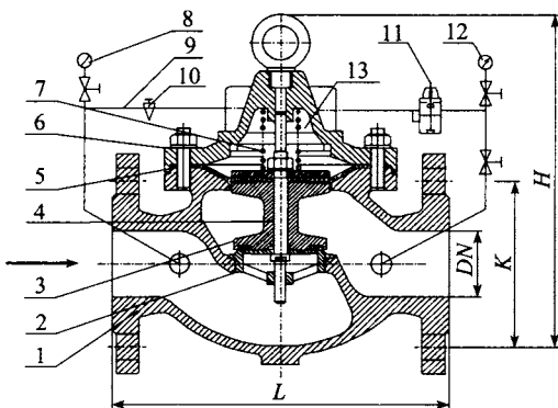
图 A. 0. 2-7 先导式稳压减压阀结构示意(卧式)
